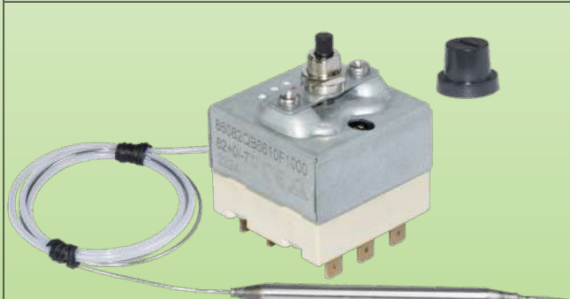
Тип с креплением при помощи центральной втулки M10
